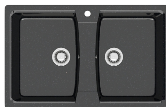
Z26 Размеры 780×500×190 мм
